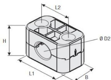
Zur Verwendung mit Kompaktschläuchen (Obere Schellenhälfte um 180° gedreht)
