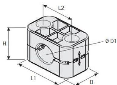
Zur Verwendung mit regulären Schläuchen
